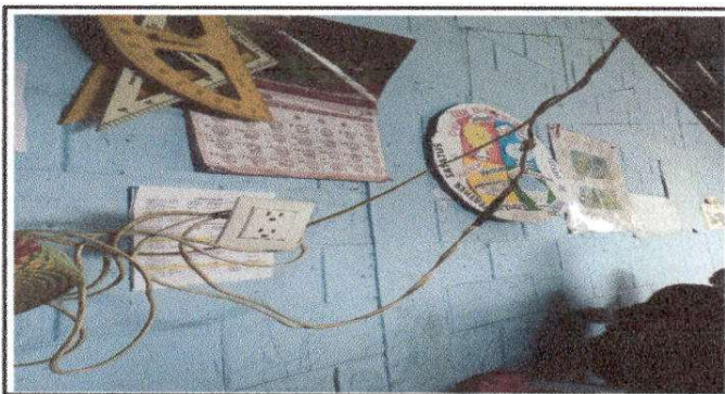
Foto 5: Sustitución de tomacorrientes dobles renglón 17.8
